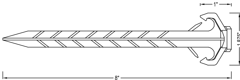
FRONT VIEW 8" 300 PCS PER CASE 70 CASES PER PALLET
